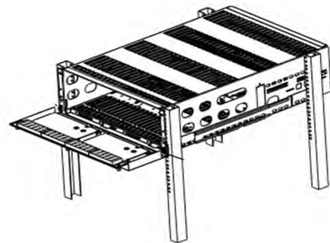
Chasis Metálico para montaje de tarjetas para System V
